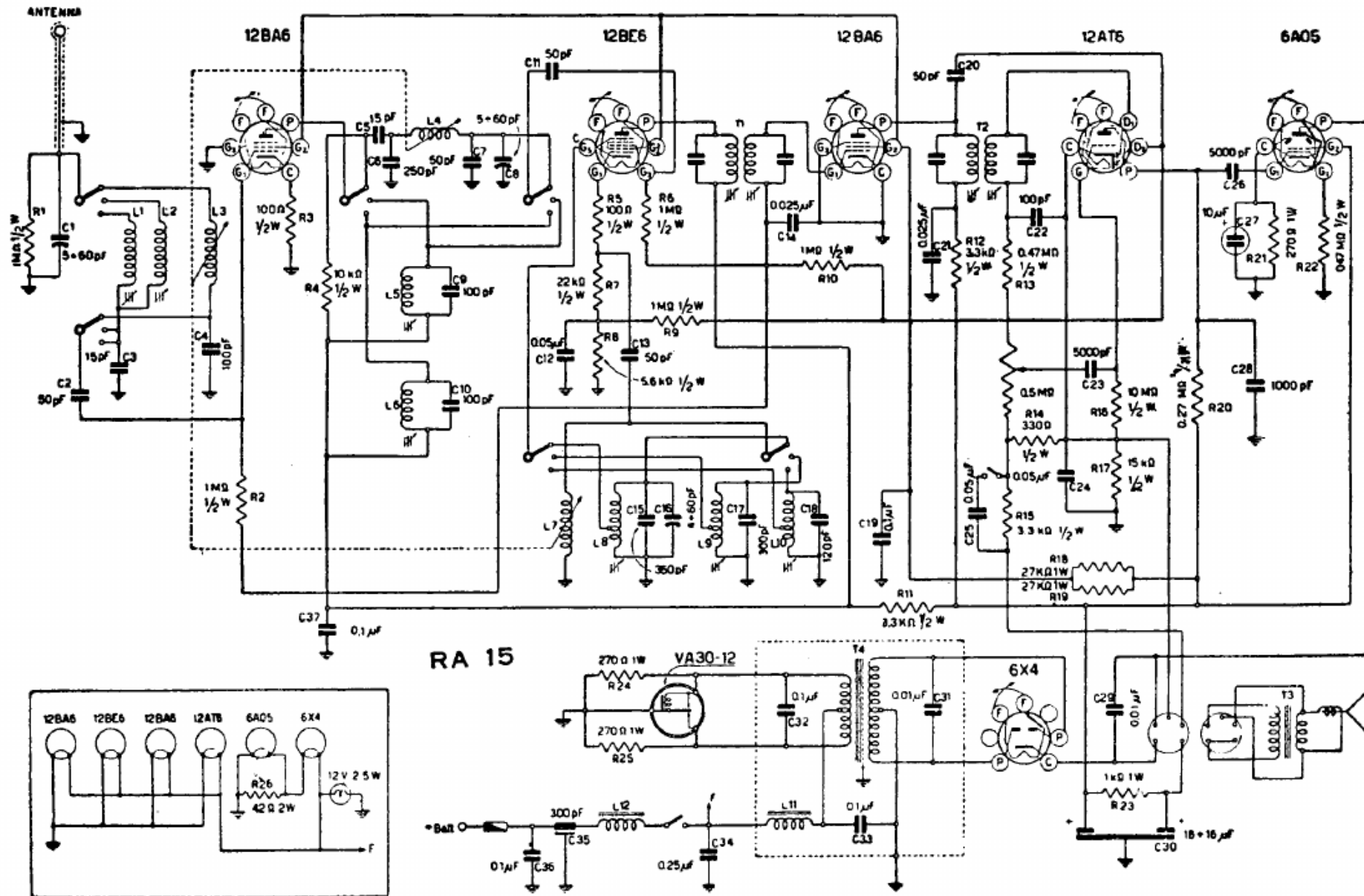
AUTOVOX - Autoradio mod. Autovox RA15. Onde medie da 520 a 1600 kc. Onde corte da 5,95 a 6,3 Mc. e da 11,7 a 12,2 Mc. Sintonia a permeabilità variabile. Media frequenza 455 kc. Consumo 3 A a 12 volt.
